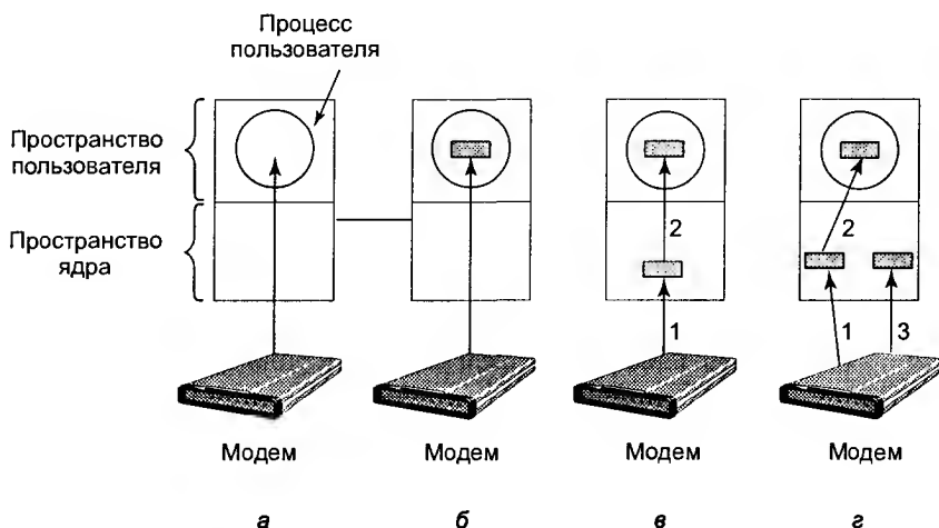
Рис. 5.11. Небуферизированный ввод (а); буферизация в пространстве пользователя (б); буферизация в ядре с копированием в пространство пользователя (в); двойная буферизация в ядре (г)
