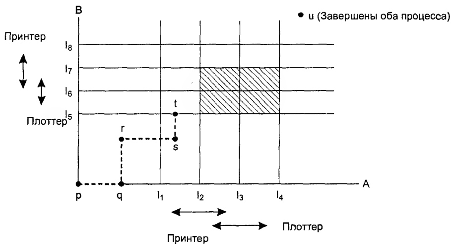
Рис. 3.6. Две траектории ресурсов процессов
