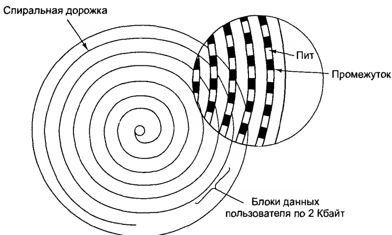
Рис. 5.16. Структура записи компакт-диска или CD-ROM
