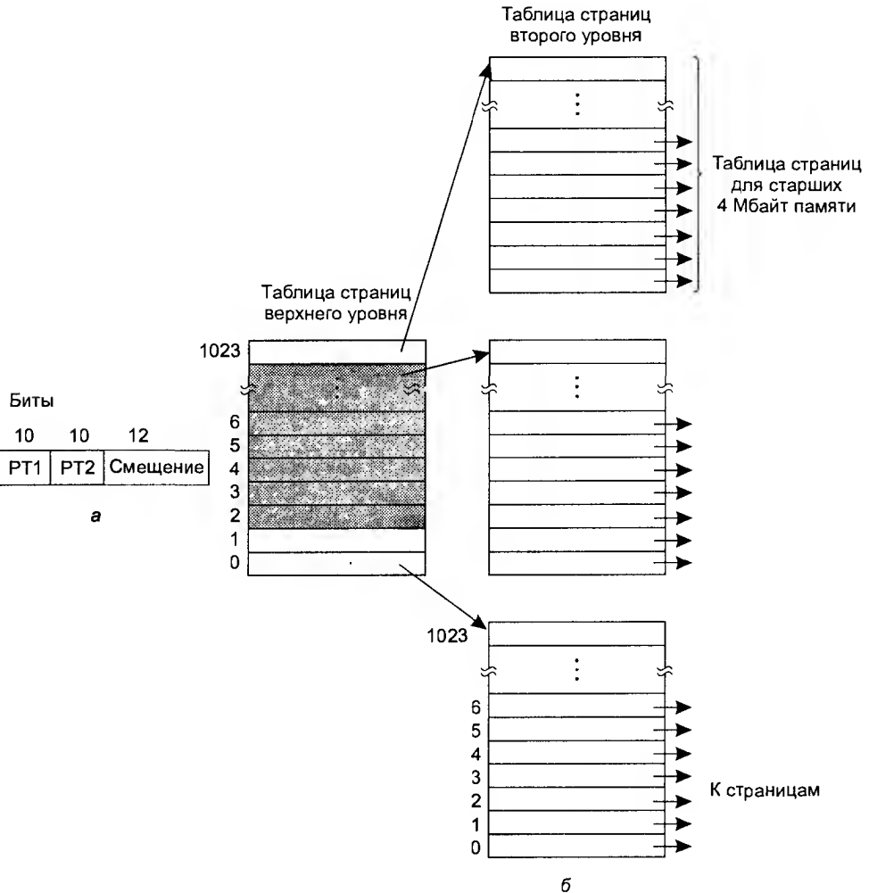
Рис. 4.12. 32-разрядные адреса с полями двух таблиц страниц (а); двухуровневая таблица страниц (б)
