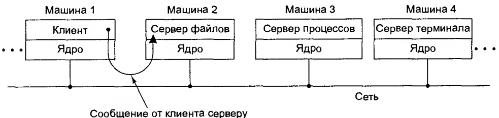
Рис. 1.24. Модель клиент-сервер в распределенной системе
