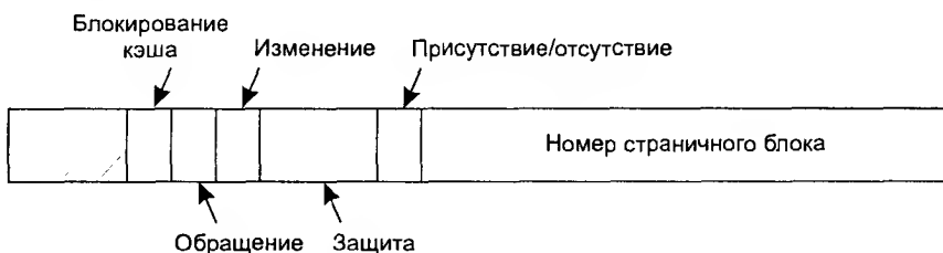
Рис. 4.13. Типичная запись в таблице страниц
