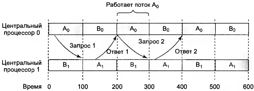
Рис. 8.14. Общение двух работающих в противофазе потоков, принадлежащих процессу A
