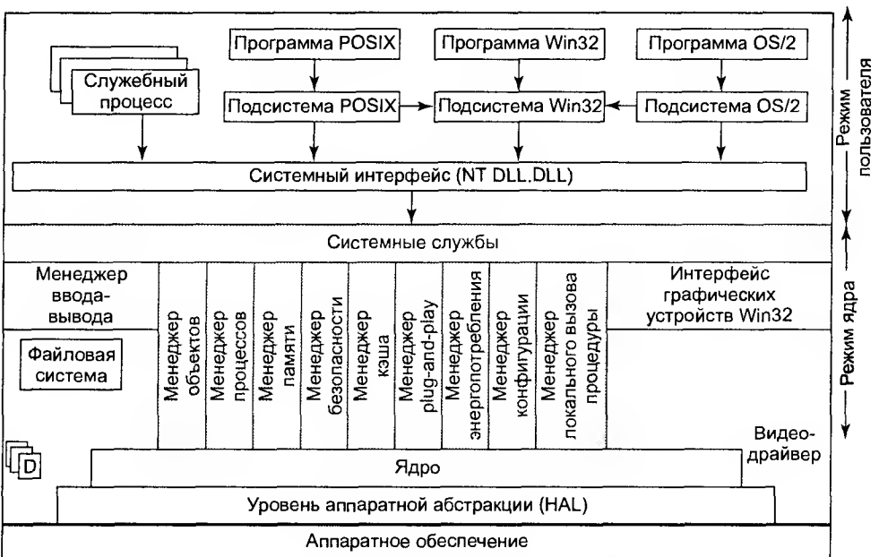
Рис. 11.2. Структура Windows 2000 (слегка упрощенная)
