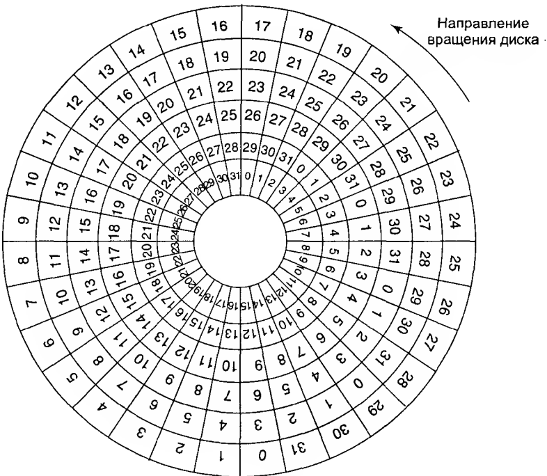
Рис. 5.21. Иллюстрация перекоса цилиндров
