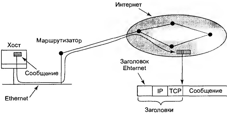
Рис. 8.31. Накапливание заголовков пакета
