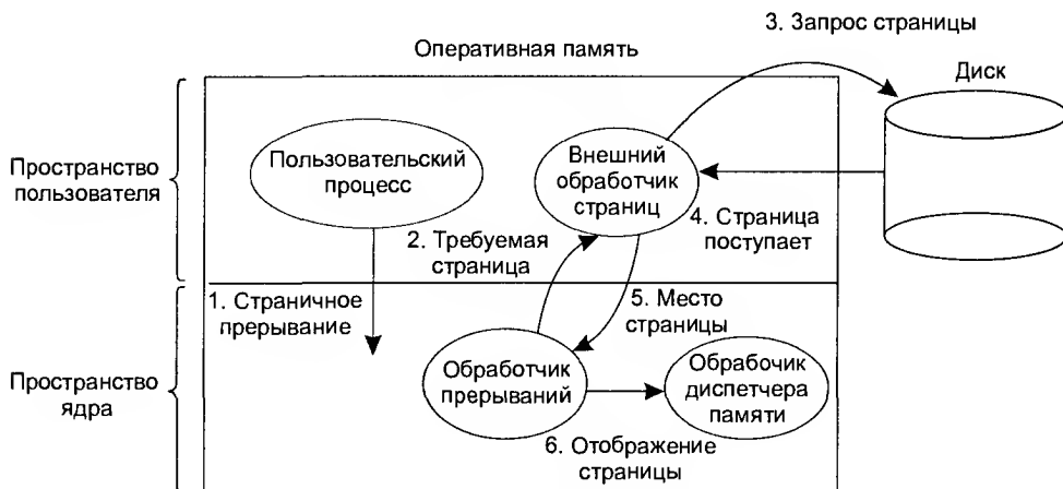
Рис. 4.32. Обработка страничного прерывания с внешним обработчиком страниц
