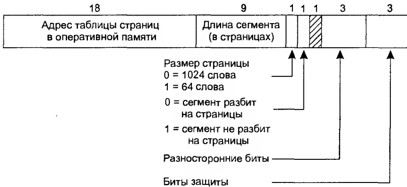
Рис. 4.36. Виртуальная память системы MULTICS: сегмент дескрипторов указывает на таблицы страниц (а); дескриптор сегмента (б). Числа означают длину полей
