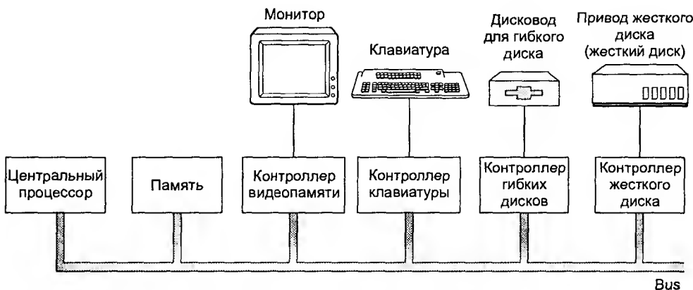
Рис. 1.5. Некоторые компоненты персонального компьютера
