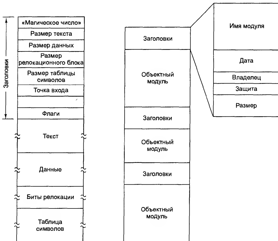
Рис. 6.2. Исполняемый файл (а); архив (б)
