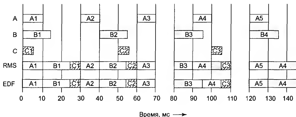
Рис. 7.11. Пример алгоритмов планирования реального времени RMS и EDF
