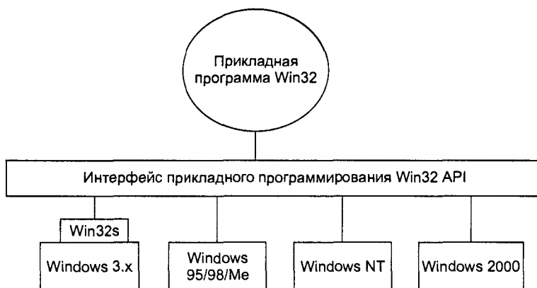
Рис. 11.1. Интерфейс Win32 API позволяет программам работать почти на всех версиях Windows
