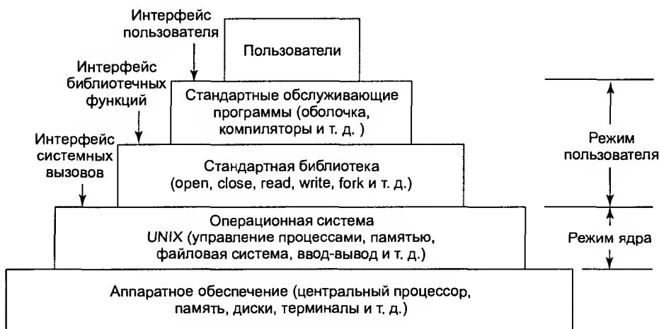
Рис. 10.1. Уровни операционной системы UNIX
