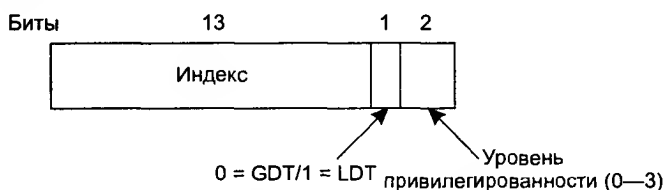
Рис. 4.40. Селектор в системе Pentium
