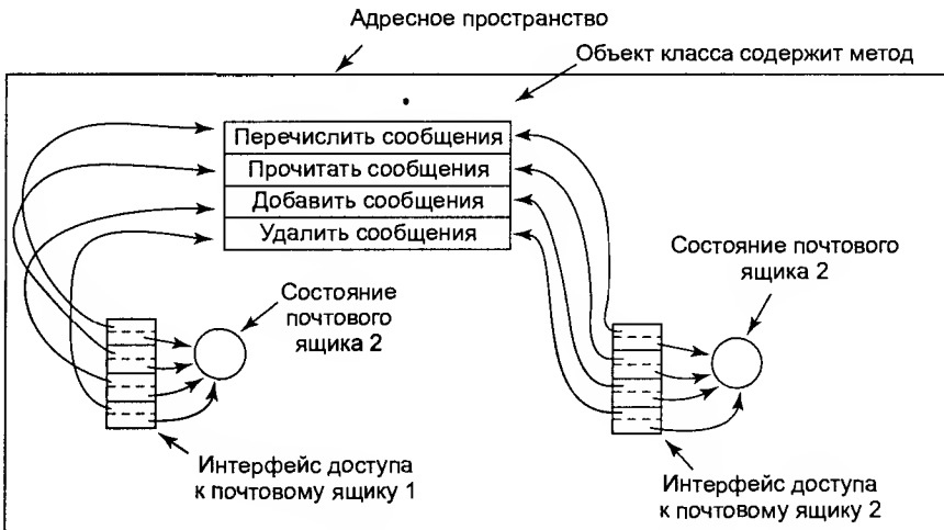
Рис. 8.38. Структура объекта Globe
