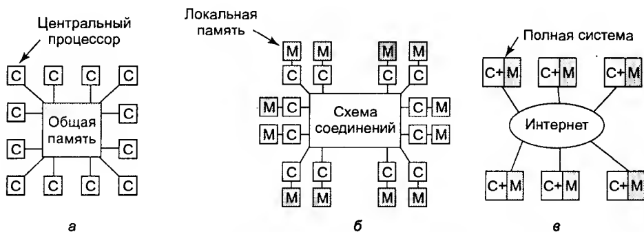
Рис. 8.1. Мультипроцессорная система с общей памятью (а); мультипроцессорная система с передачей сообщений (б); глобальная распределенная система (в)
