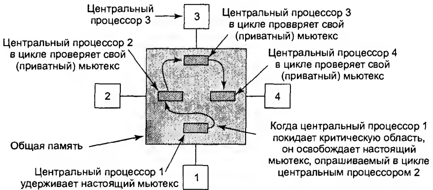
Рис. 8.11. Использование нескольких мьютексов во избежание пробуксовки кэша
