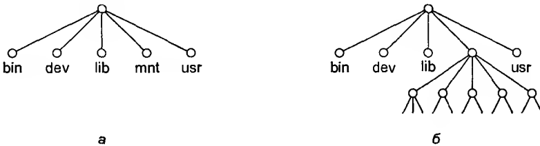
Рис. 1.19. Два каталога до присоединения /usr/jim/memo к каталогу ast (а); те же каталоги после вызова link (б)
