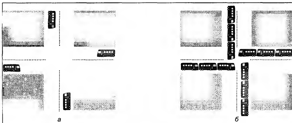
Рис. 1.13. Потенциальная взаимоблокировка (а); фактическая взаимоблокировка (б)
