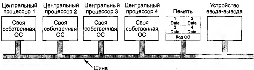
Рис. 8.7. Разделение памяти мультипроцессора между четырьмя центральными процессорами с общей копией кода операционной системы
