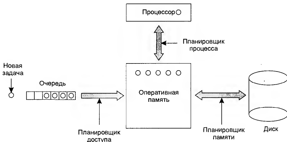
Рис. 2.22. Трехуровневое планирование
