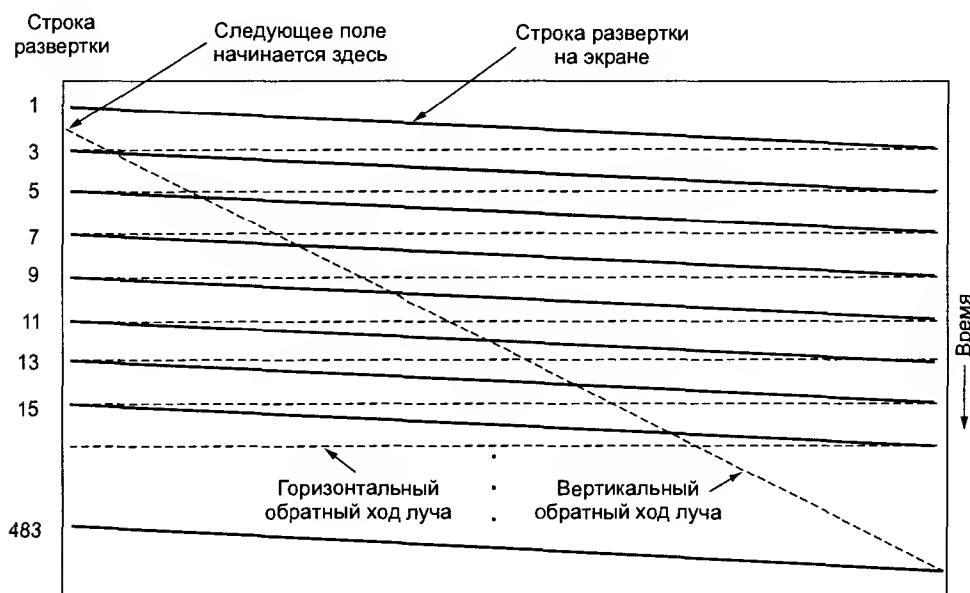
Рис. 7.4. Путь сканирующего луча в видеосистеме NTSC
