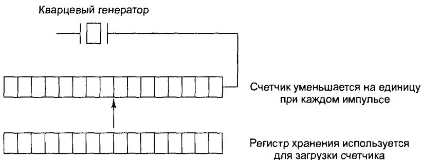
Рис. 5.27. Программируемый таймер
