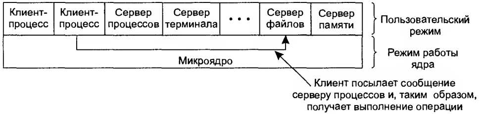
Рис. 1.23. Модель клиент-сервер
