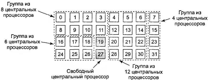
Рис. 8.13. Набор из 32 центральных процессоров, разделенный на четыре группы, плюс два процессора свободны
