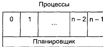
Рис. 2.3. Нижний уровень операционной системы отвечает за прерывания и планирование. Выше расположены последовательные процессы
