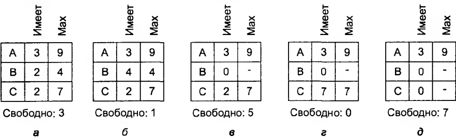
Рис. 3.7. Демонстрация того, что состояние a безопасно
