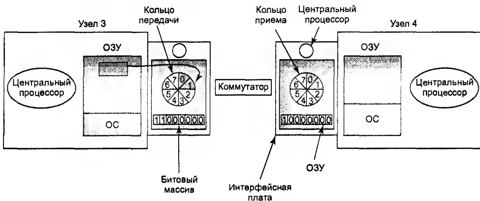
Рис. 8.19. Использование колец передачи и приема для координации центрального процессора с процессором на плате
