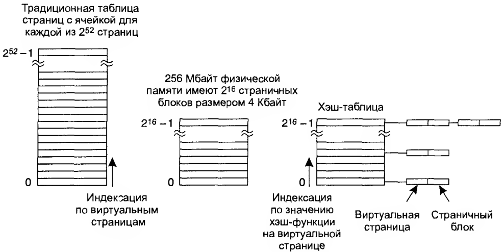
Рис. 4.14. Сравнение традиционной таблицы страниц с инвертированной
