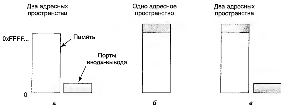
Рис. 5.1. Раздельные адресные пространства (а); отображаемый на адресное пространство памяти ввод-вывод (б); гибрид (в)
