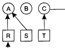
Рис. 3.2. Пример возникновения взаимоблокировки и способы избежать ее
