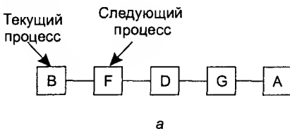
Рис. 2.23. Циклическое планирование: список процессов в состоянии готовности (а); список процессов в состоянии готовности после того, как процесс В исчерпал свой квант времени (б)
