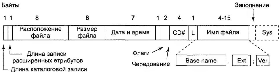
Рис. 6.26. Каталогная запись стандарта ISO 9660
