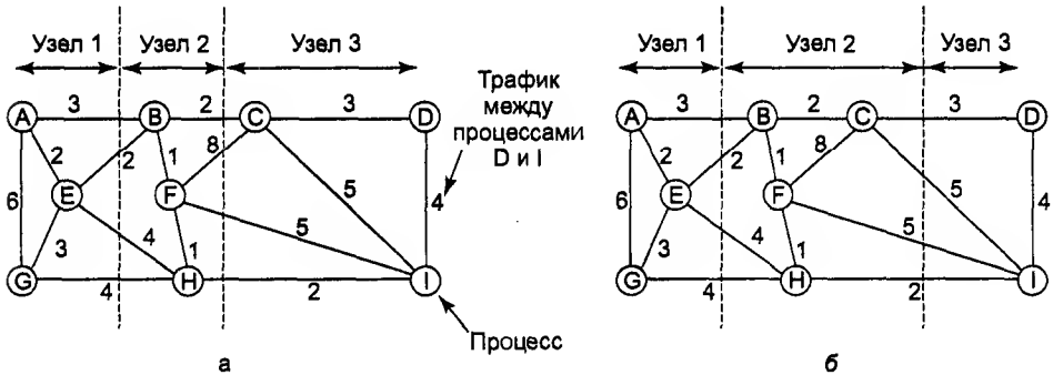
Рис. 8.25. Два способа распределения девяти процессов на трех узлах
