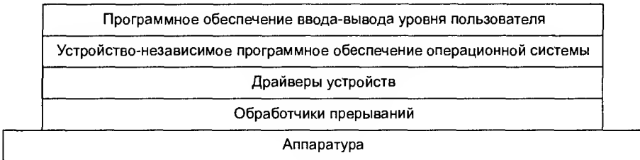
Рис. 5.8. Программные уровни ввода-вывода
