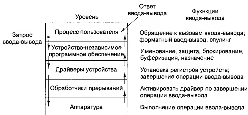
Рис. 5.13. Уровни и основные функции системы ввода-вывода
