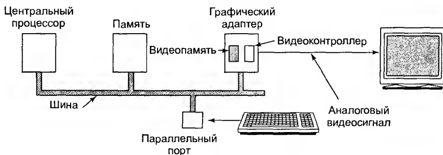
Рис. 5.32. Дисплей с общей памятью
