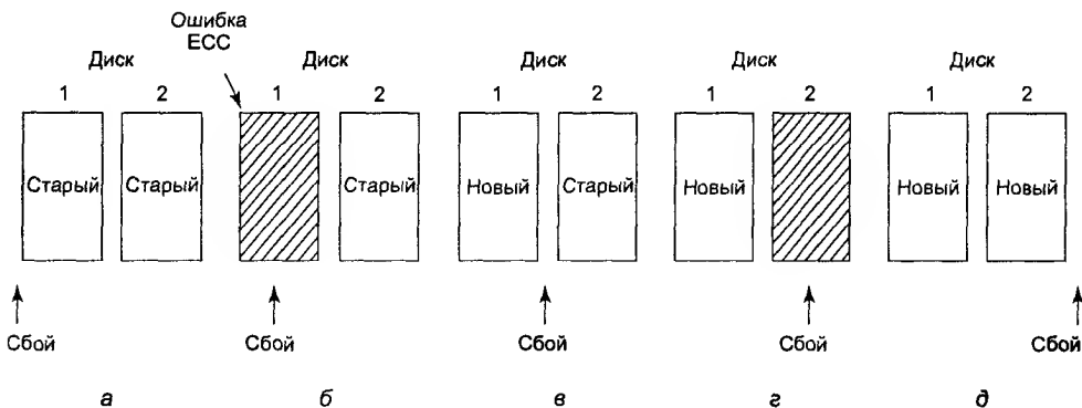
Рис. 5.26. Анализ влияния сбоя процессора на стабильность записи
