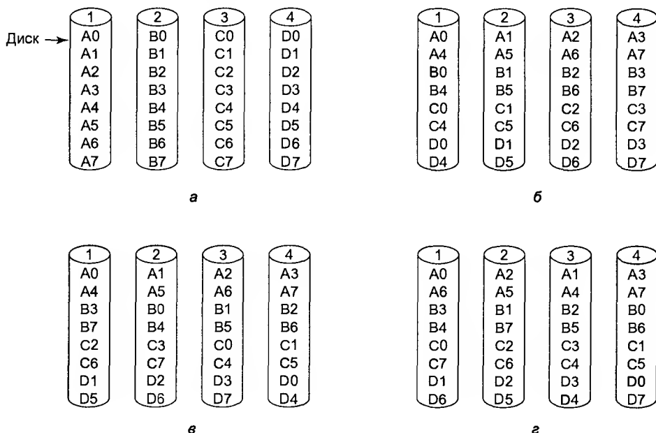
Рис. 7.21. Четыре способа организации мультимедийных файлов на нескольких дисках: без чередования (а); с одинаковым чередованием для всех файлов (б); в шахматном порядке (в); со случайным чередованием (г)
