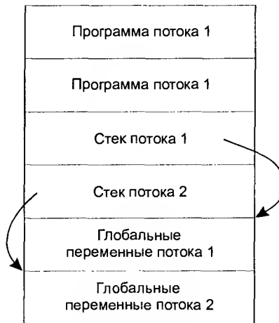
Рис. 2.13. У потоков могут быть собственные глобальные переменные
