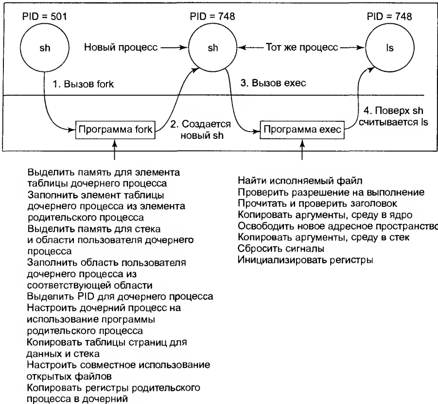
Рис. 10.3. Этапы выполнения команды ls , введенной в оболочке
