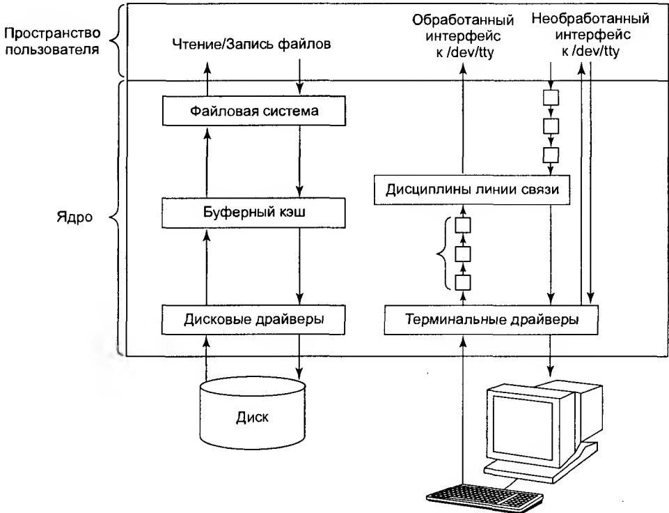
Рис. 10.12. Система ввода-вывода BSD UNIX
