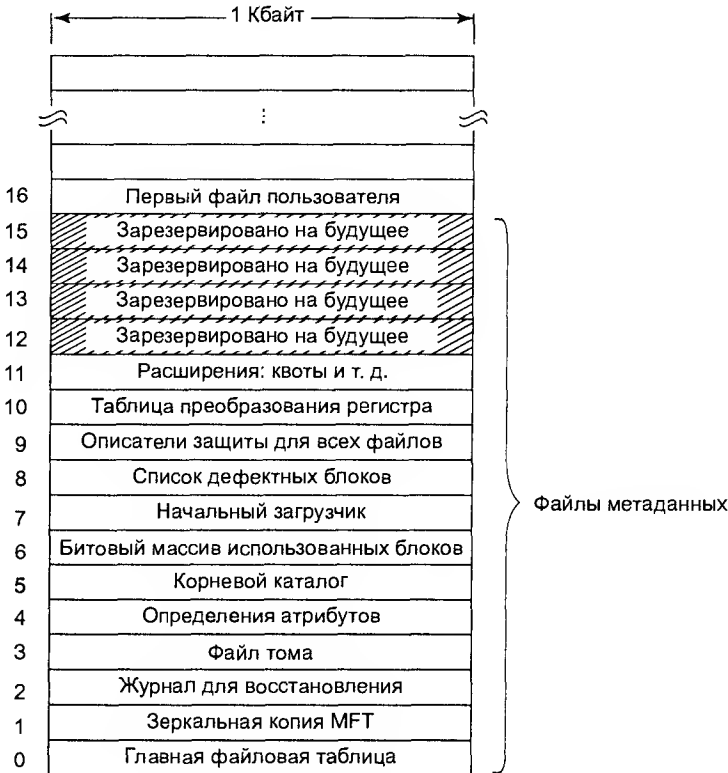
Рис. 11.17. Главная файловая таблица NTFS
