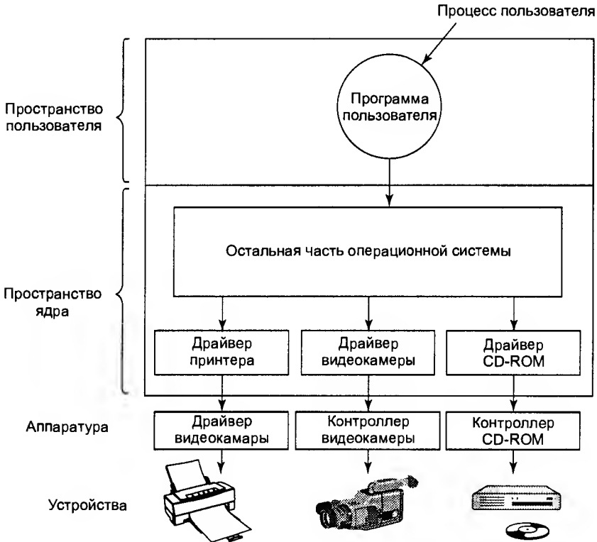
Рис. 5.9. Логическое расположение драйверов устройств. На самом деле весь обмен информацией между драйверами и контроллерами устройств идет по шине
