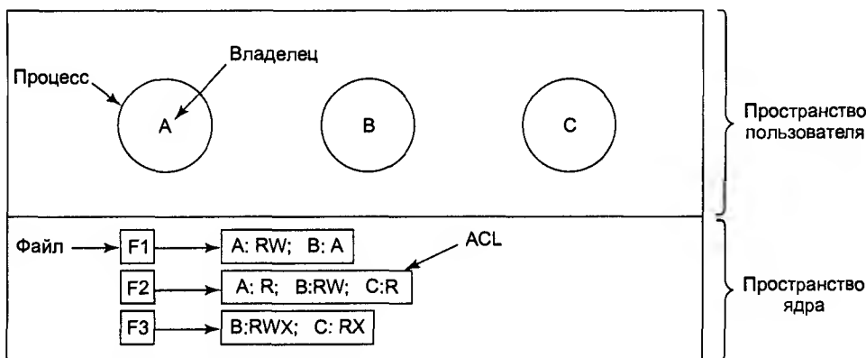
Рис. 9.17. Использование ACL-списков для управления доступом к файлам
