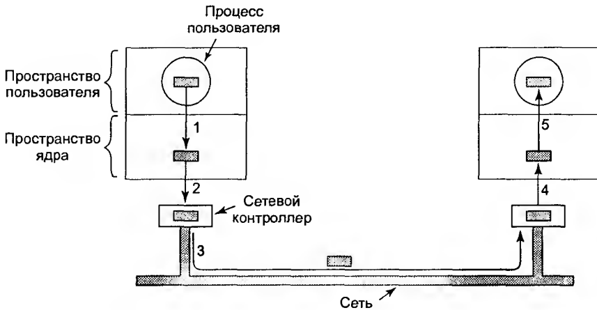
Рис. 5.12. Копии пакета при передаче его по сети
