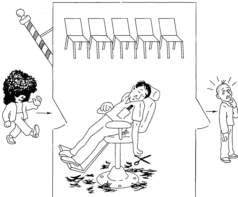
Рис. 2.19. Спящий брадобрель
