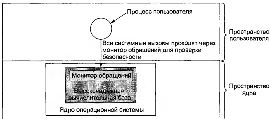
Рис. 9.20. Монитор обращений
