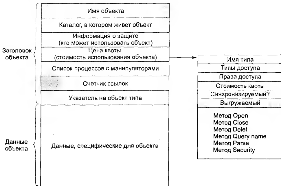
Рис. 11.4. Структура объекта
