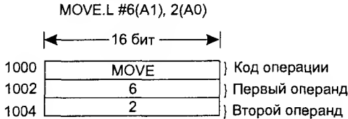
Рис. 4.30. Команда, вызвавшая страничное прерывание
