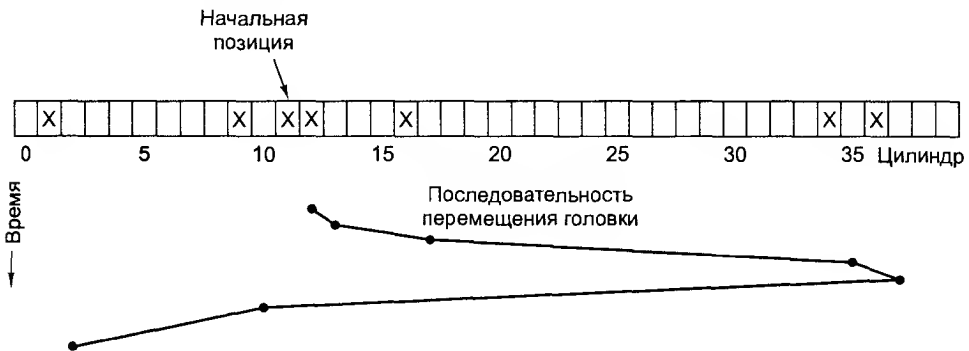
Рис. 5.24. Элеваторный алгоритм планирования обращений к диску
