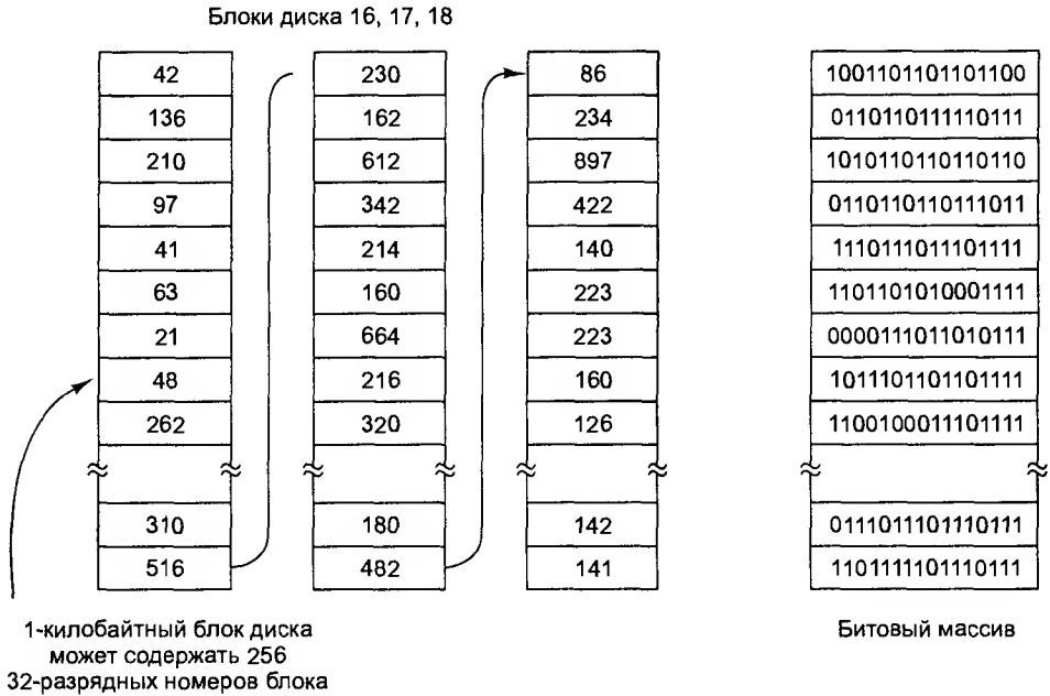
Рис. 6.18. Хранение информации о свободных блоках в виде списка (а); битовый массив (б)
