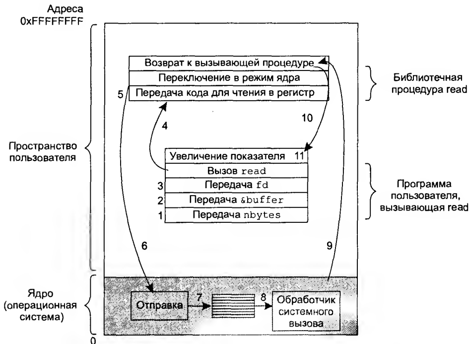
Рис. 1.17. 11 шагов выполнения системного вызова read(fd, buffer, nbytes)
