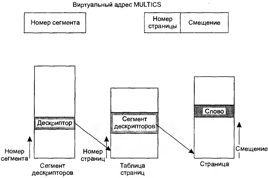
Рис. 4.38. Преобразование в системе MULTICS адреса, состоящего из двух частей, в адрес в оперативной памяти
