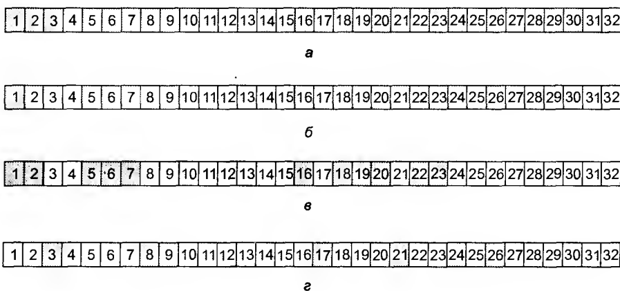
Рис. 6.22. Битовые массивы, используемые алгоритмом логической архивации
