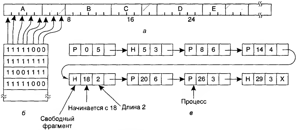
Рис. 4.7. Часть памяти с пятью процессами и тремя свободными областями (а); соответствующая битовая карта (б); та же информация в виде списка (в)
