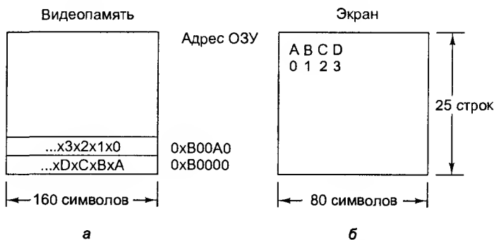
Рис. 5.33. Видеопамять монохромного дисплея, работающего в символьном виде (а); соответствующий экран (б). Символами \times обозначены байты атрибутов
