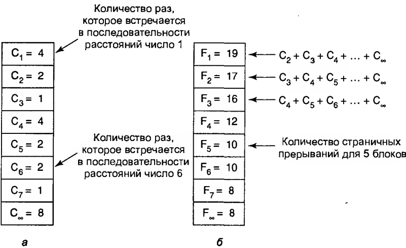
Рис. 4.25. Вычисление количества страничных прерываний из последовательности расстояний: вектор C (а); вектор F (б)
