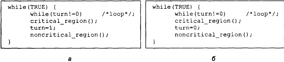
Рис. 2.16. Предлагаемое решение проблемы критической области: процесс 0 (а); процесс 1 (б). В обоих случаях необходимо удостовериться в наличии точки с запятой, ограничивающей цикл while
