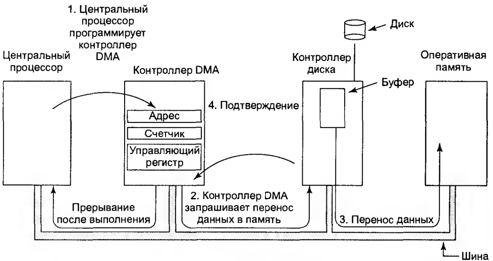
Рис. 5.3. Работа DMA-контроллера
