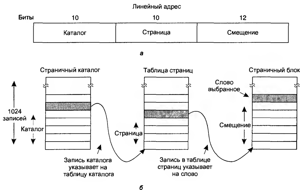
Рис. 4.43. Отображение линейного адреса на физический адрес
