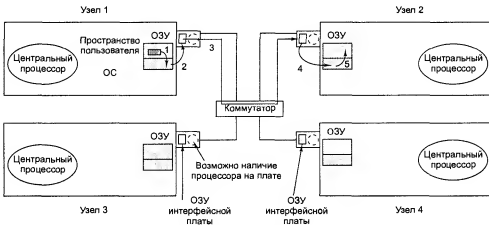
Рис. 8.18. Расположение сетевых интерфейсных плат в мультимедийном компьютере
