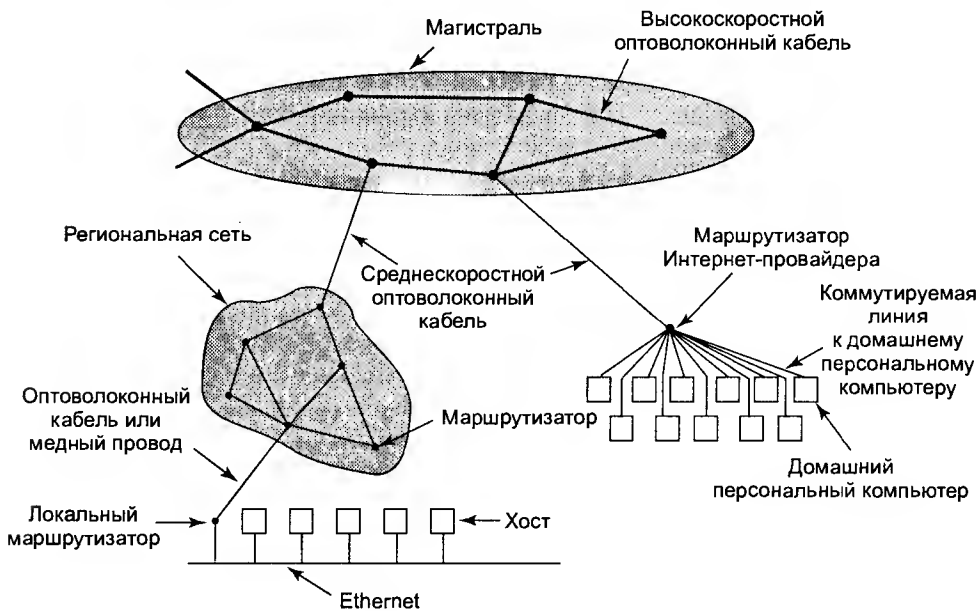
Рис. 8.29. Часть Интернета
