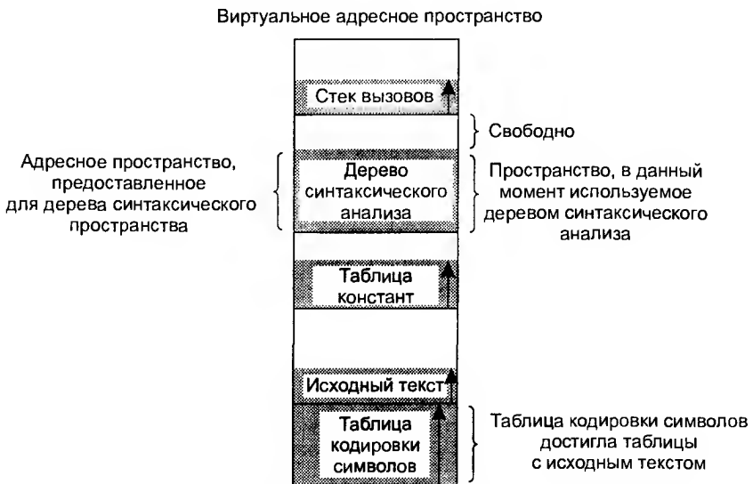
Рис. 4.33. В одномерном адресном пространстве при росте таблиц одна может упереться в другую
