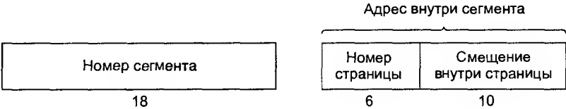
Рис. 4.37. 34-разрядный виртуальный адрес в системе MULTICS
