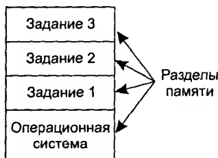
Рис. 1.4. Многозадачная система с тремя заданиями в памяти
