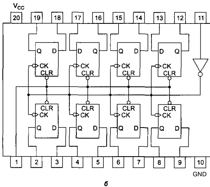
Рис. 3.27. Два D-триггера (а); восьмиразрядный триггер (б)
