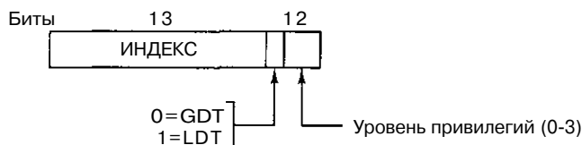
Рис. 6.10. Селектор в машине Pentium II
