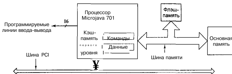
Рис. 3.45. Система microjava II 701
