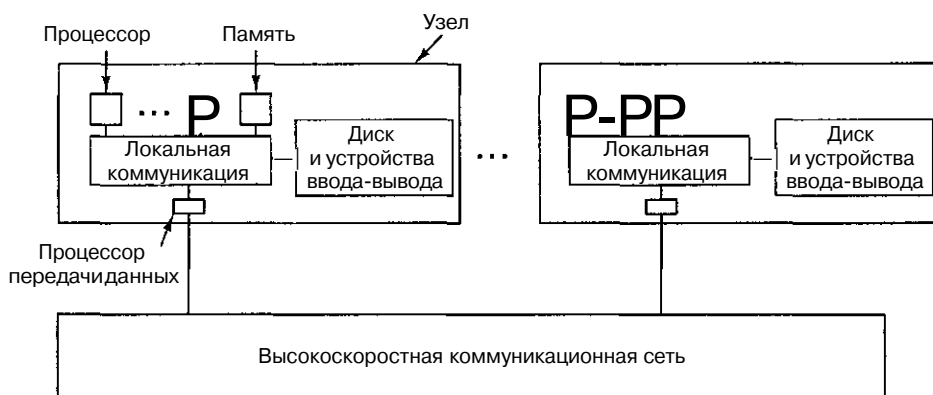
Рис. 8.28. Схема мультимышьятера
