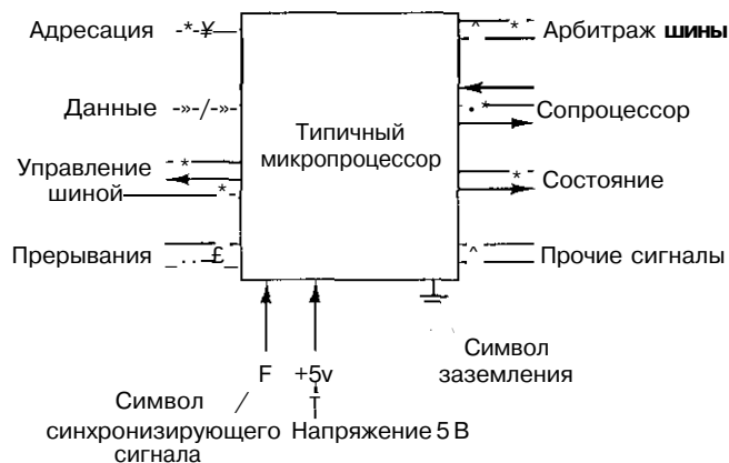
Рис. 3.31 . Цоколевка типичного центрального процессора. Стрелочки указывают входные и выходные сигналы. Короткие диагональные линии указывают на наличие нескольких выводов. Для конкретных процессоров будет дано число этих выводов
