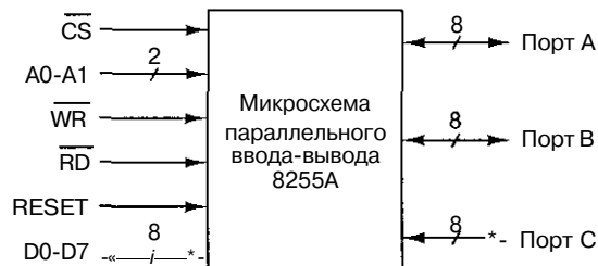
Рис. 3. 51. Микросхема 8255А
