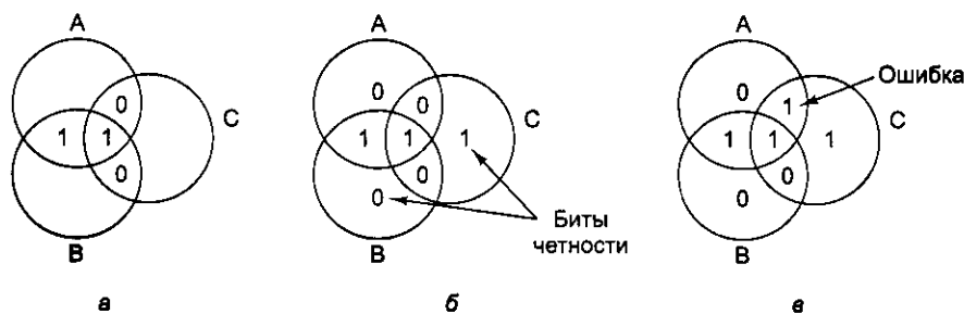
Рис. 2.11. Кодировка числа 1100 (а); добавляются биты четности (б); ошибка в секторе АС (в)
