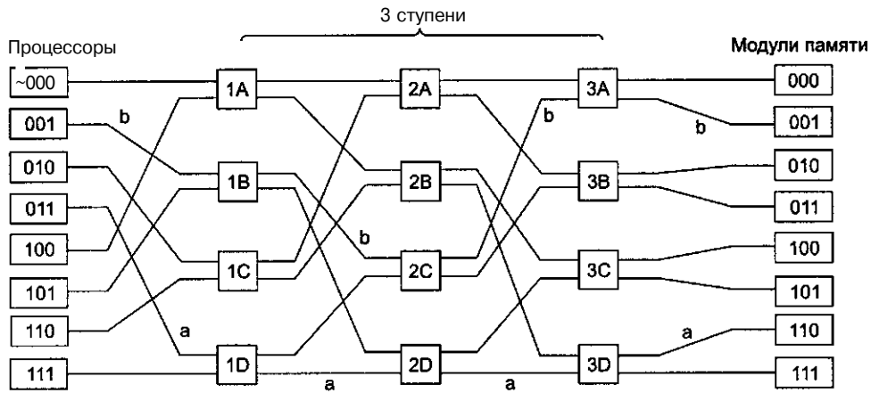
Рис. 8.22. Сеть омега
