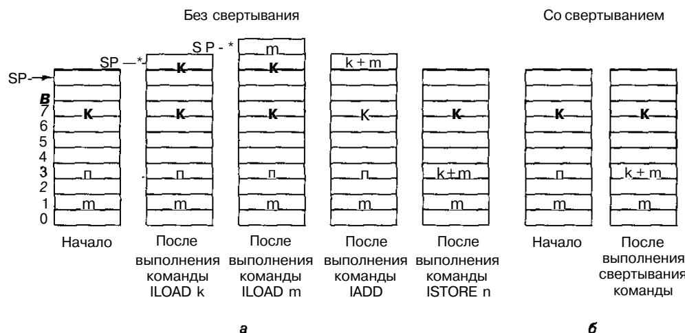
Рис. 4.38. Выполнение последовательности из четырех команд для вычисления выражения n = k + m (а); также последовательность, свернутая до одной команды (б)
