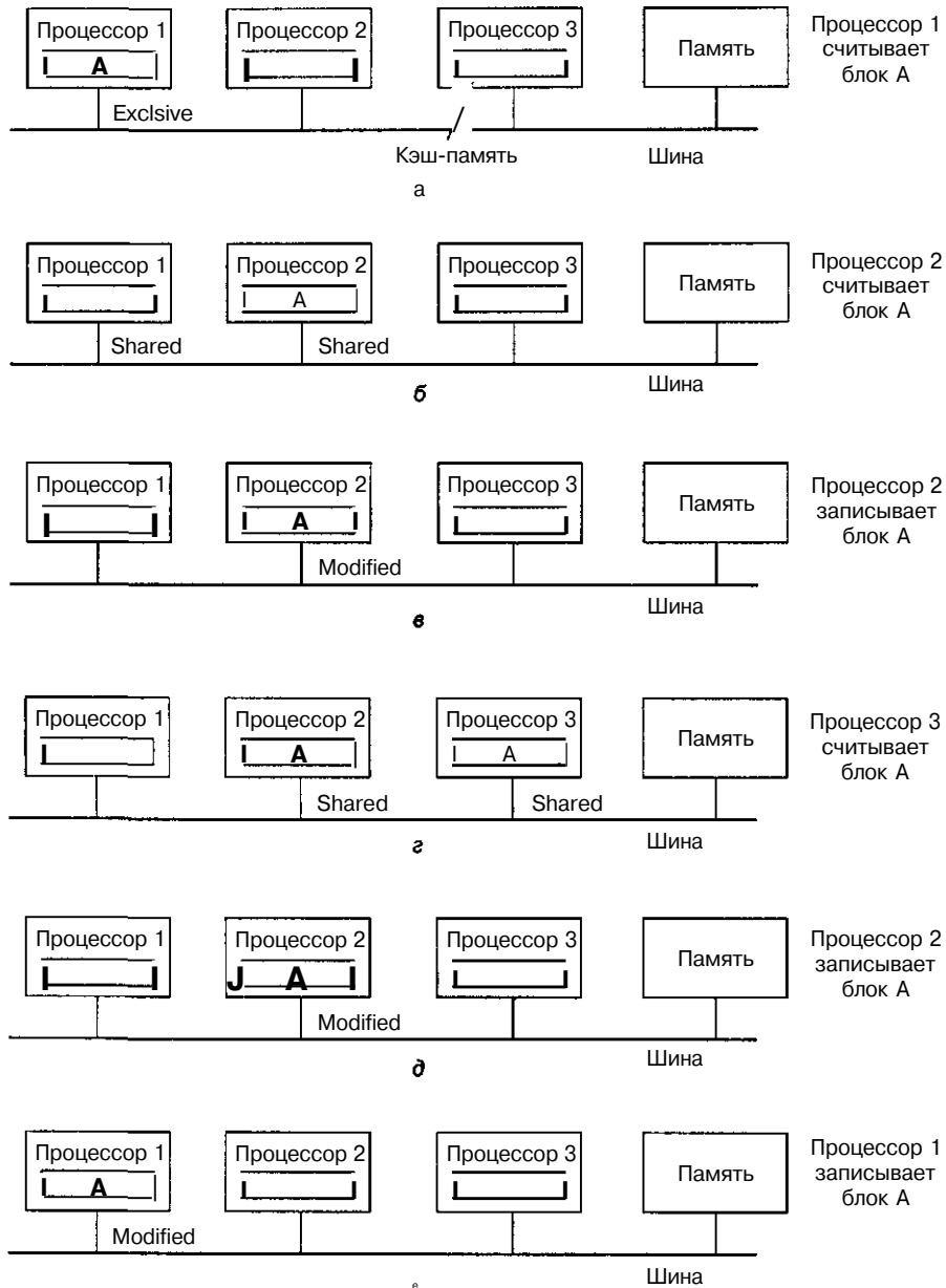
Рис. 8.18. Протокол MESI
