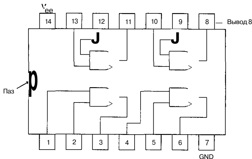
Рис. 3.9. Микросхема МИС, содержащая 4 вентиля
