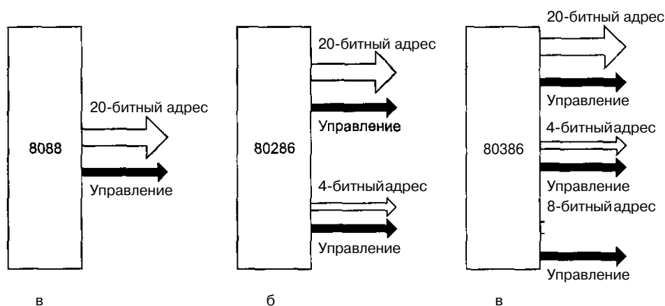
Рис. 3.33. Расширение адресной шины течением времени
