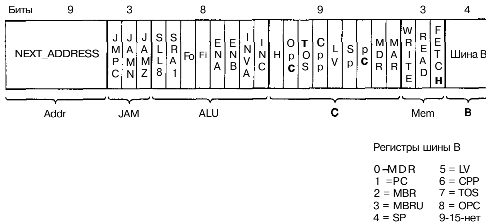
Рис. 4.4. Формат микрокоманды для Мю-1
