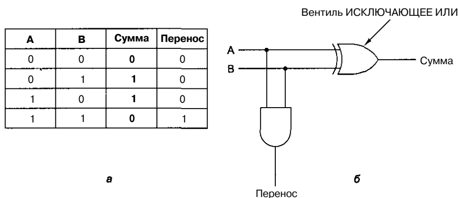
Рис. 3.16. Таблица истинности для сложения одnorазрядных чисел (а); схема полусумматора (б)
