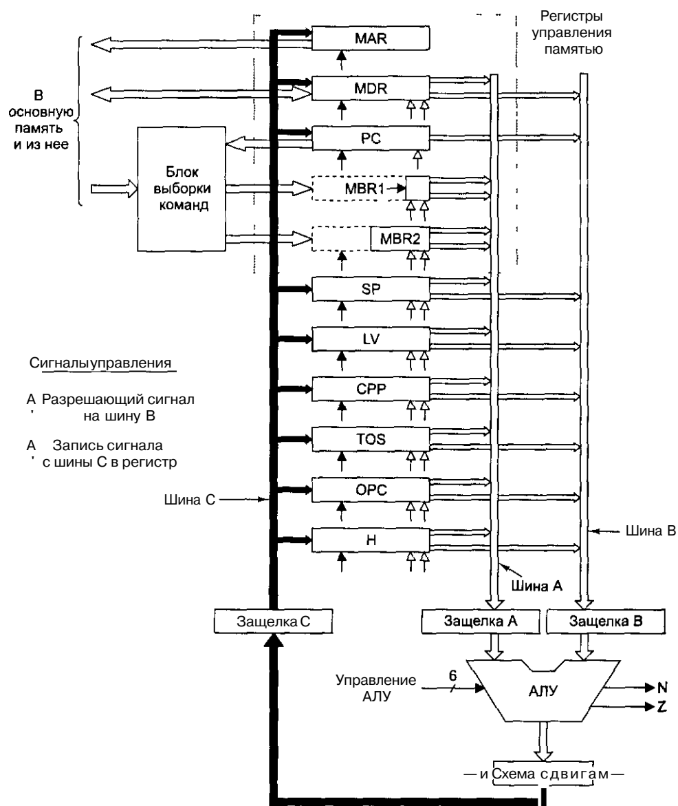
Рис. 4.21, Трассировка шин в микроархитектуре Mic-3
