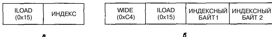
Рис. 4.14. Команда ILOAD с одnobайтным индексом (а); команда WIDE ILOAD с двубайтным индексом (б)
