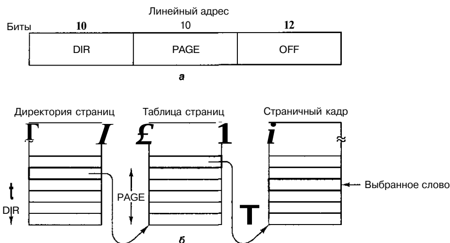
Рис. 6.13. Отображение линейного адреса на физический адрес
