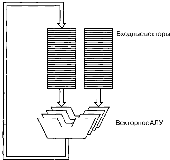
Рис. 8.13. Векторное АЛУ
