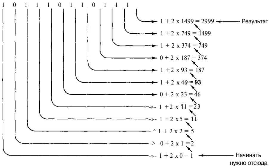
Рис. А.5. Преобразование двоичного числа 1011101011 в десятичное путем последовательного удваивания снизу вверх. В каждой следующей строке удваивается значение предыдущей строки и прибавляется соответствующий бит. Например, 374 умножается на 2 и прибавляется бит соответствующей строки (в данном случае 1). В результате получается 749
