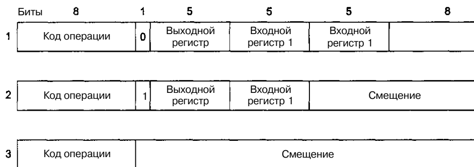
Рис. 5.16. Разработка форматов команд для трехадресной машины
