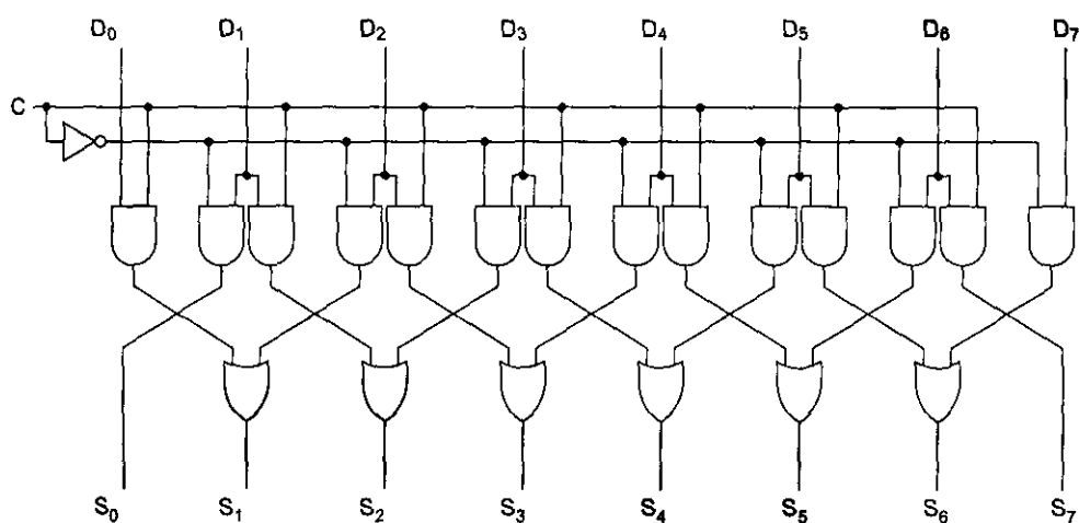
Рис. 3.15. Схема сдвига
