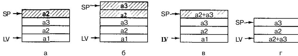
Рис. 4.8. Использование стека операндов для арифметических действий
