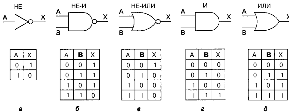
Рис. 3.2. Значки для изображения 5 основных вентилях. Поведение функции для каждого вентиля
