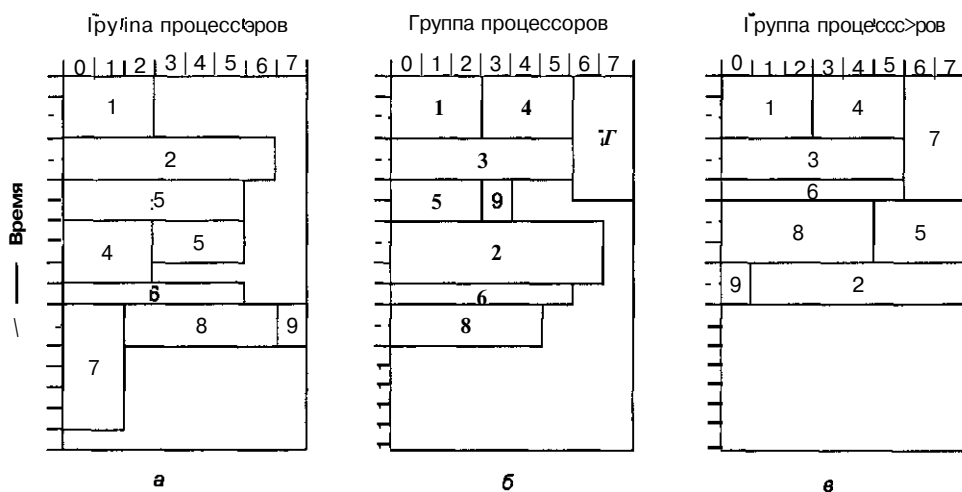
Рис. 8.31 . Планирование работы в системе COW: FIFO («первым вошел — первым вышел») (а); безблокировки начала очереди (б); заполнение прямоугольника «процессоры-время» (в). Серым цветом показаны свободные процессоры
