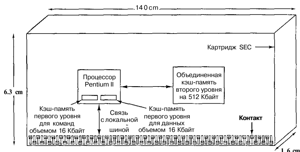
Рис. 3.40. Компонировка SEC
