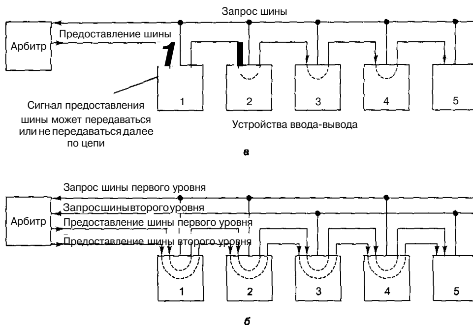
Рис. 3.36. Одноуровневый централизованный арбитраж шины с использованием системы последовательного опроса (а); двухуровневый централизованный арбитраж (б)
