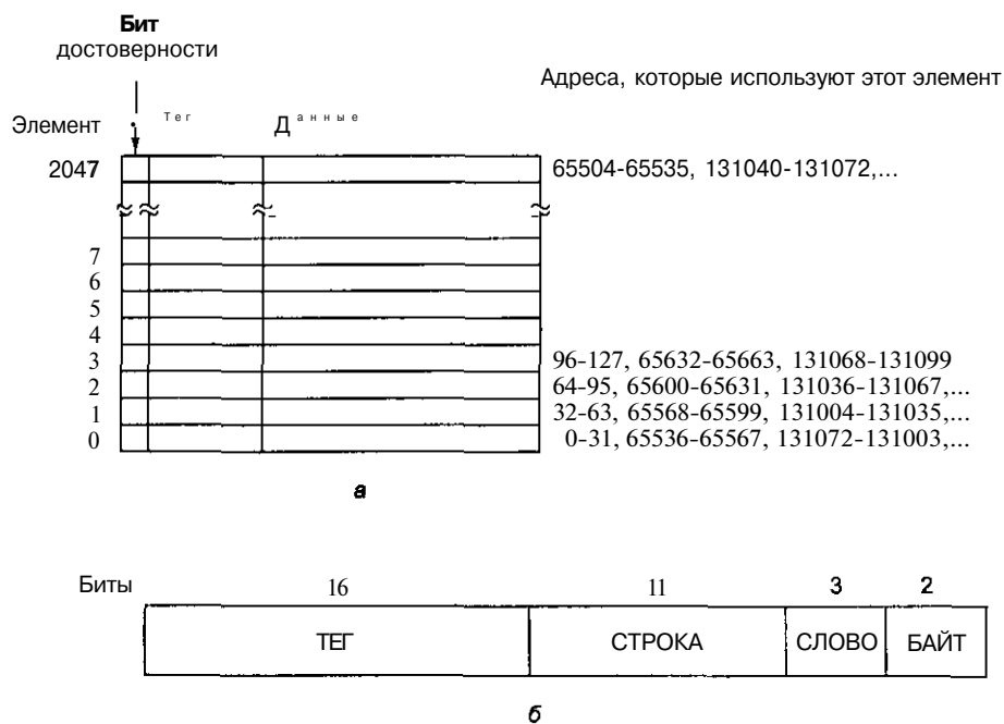
Рис. 4.26. Кэш-память прямого отображения (а); 32-битный виртуальный адрес (б)
