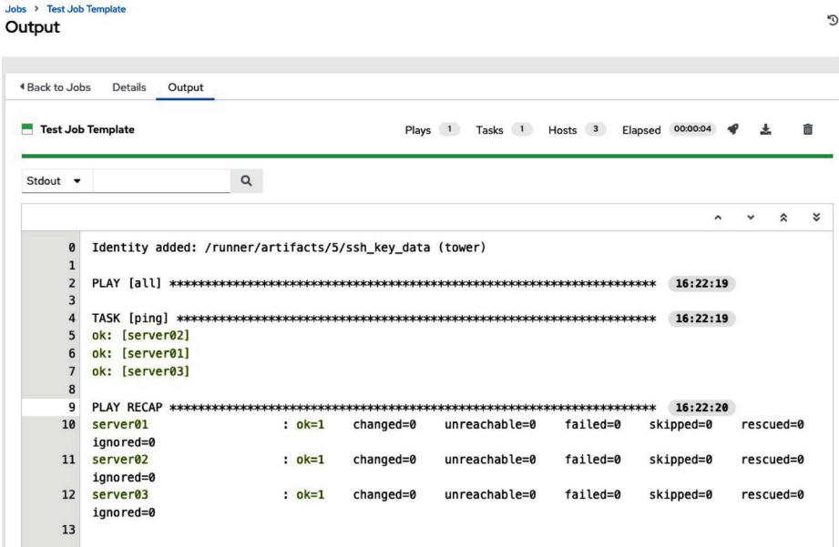
Рис. 23.12. Подробный обзор результатов задания в Ansible Automation Platform
