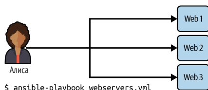
Playbook: webservers.yml
